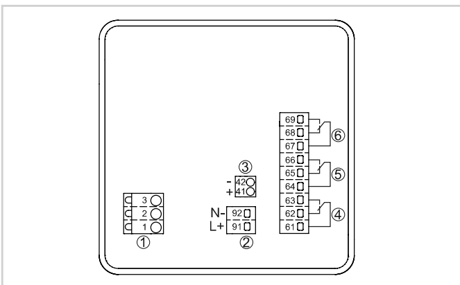
Anschlussplan VEGAMET 341
